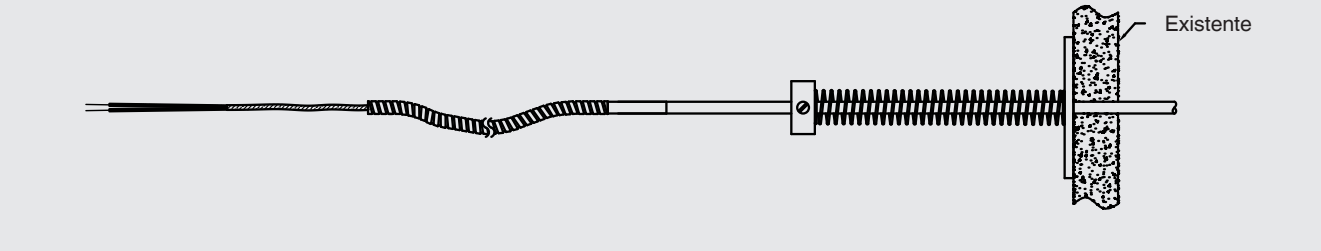
Conexión deslizante (pistón/resorte) con el horno, estilo de resorte
