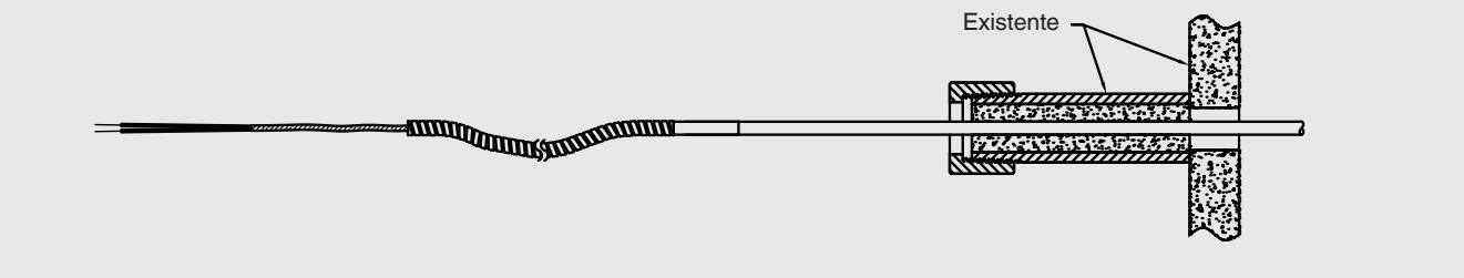
Conexión deslizante (pistón/resorte) con el horno, estilo de pistón
