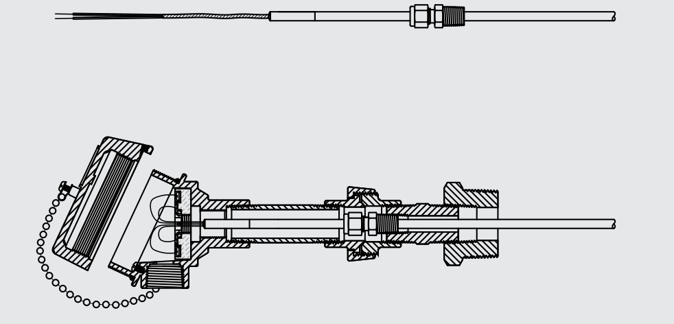
Conexión fija (racor deslizante) en el horno
